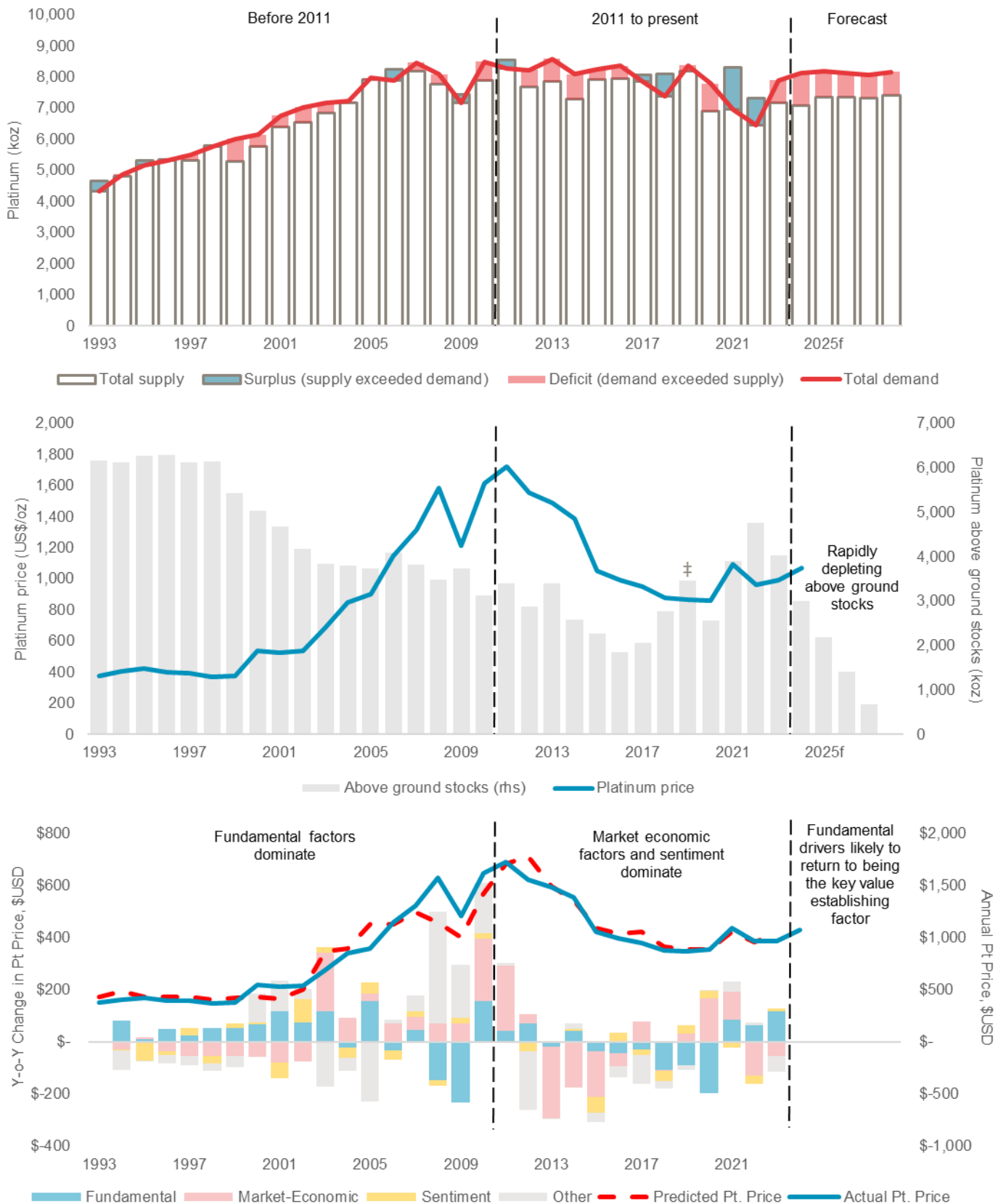
図 11.上から順に、①プラチナの需給とマーケットバランス、②プラチナの地上在庫と過去のプラチナ価格、③価格モデルが予測した過去の価格とその決定要因と実際の過去の価格。
