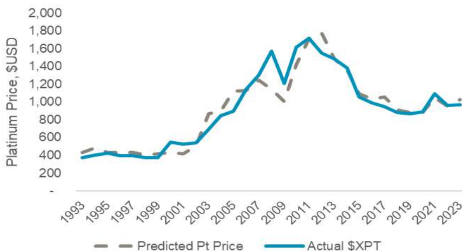
図 8. モデルを使って予測したプラチナ価格は年毎の実際のプラチナ価格に近い動きを示している。世界金融危機などその他の要因があった年(2007年~2008年)は予測と実際の価格に差がある
