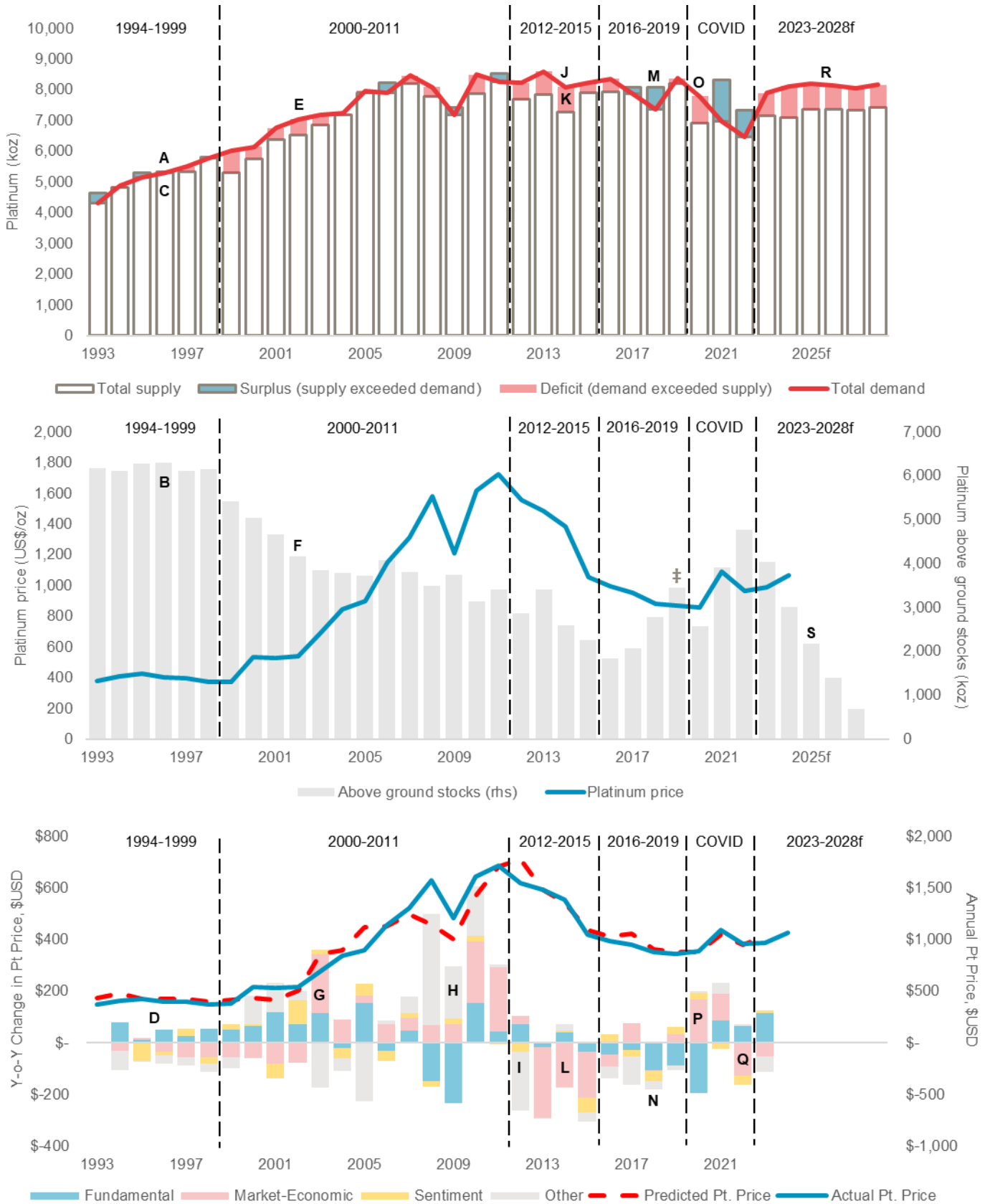
図 15. 上から順に、①プラチナの需給とマーケットバランス、②プラチナの地上在庫と過去のプラチナ価格、③価格モデルが予測した過去の価格とその決定要因と実際の過去の価格。これらのチャートは16ページ「マーケットの変遷」の記述中アルファベットの記号で指摘した箇所と合わせて考察していただきたい。
